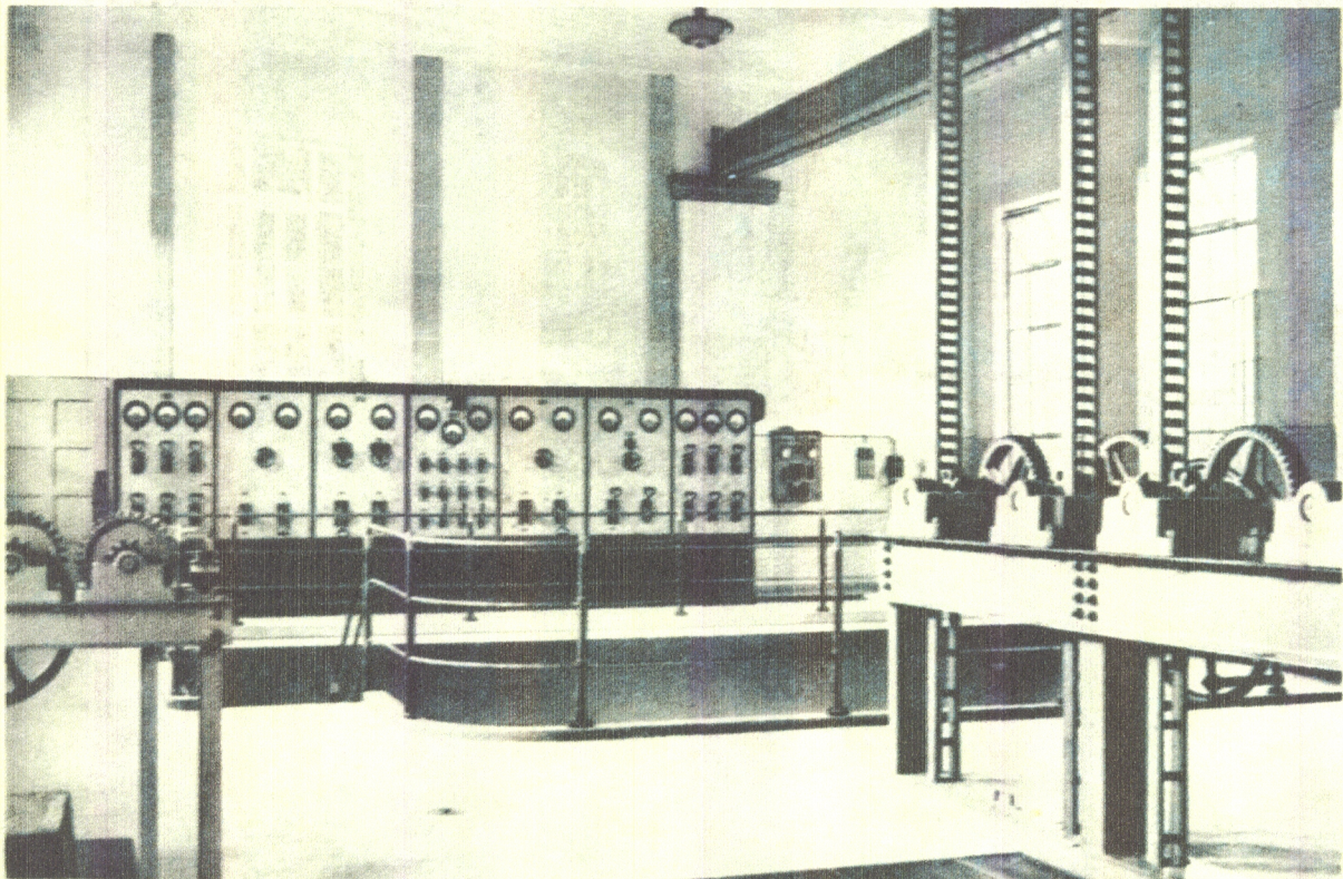
Turbinenhaus mit Schaltanlage
